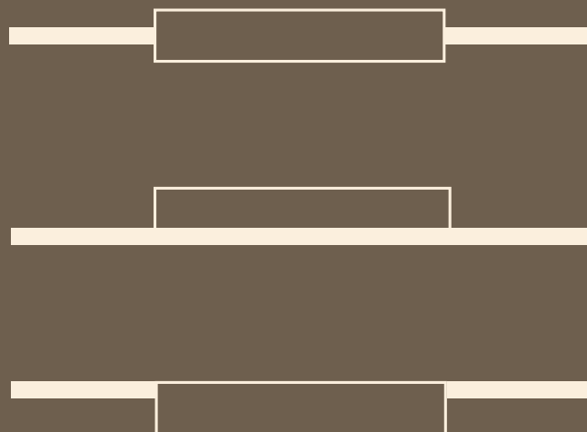
↑ Trzy dostępne warianty montażu umywarek Geberit Variform: umywalki nablatowe, wpuszczane w blat i podblatowe.
